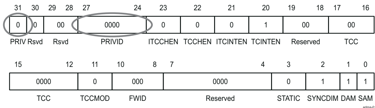
Figure 18-30. Channel Options Parameter (OPT) Example
