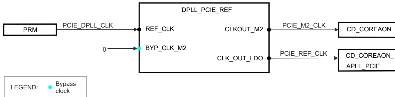
Figure 3-63. DPLL_PCIE_REF Overview
