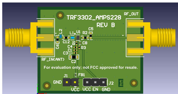
TRF3302Q1EVM Top View
