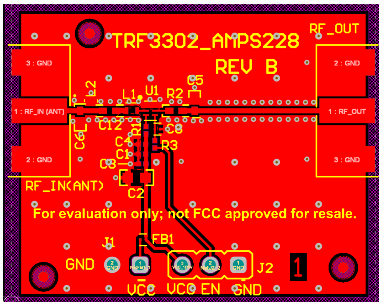
Figure 3-4. Top Layer
