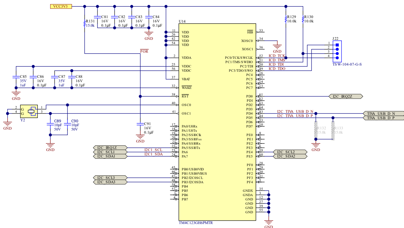
Figure 4-6. TIVA USB I2C MCU
