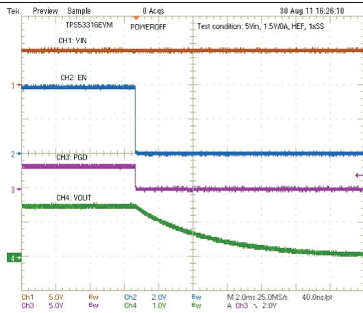
5-V VIN, 1.5-V VOUT, and 0-A IOUT
