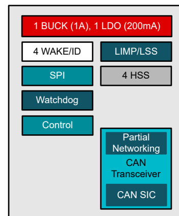
TCAN2451-Q1 Diagram
