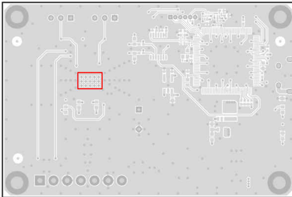
Figure 10-4. Bottom Layer
