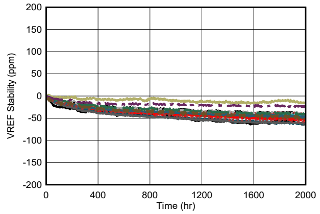
WCSP Package
