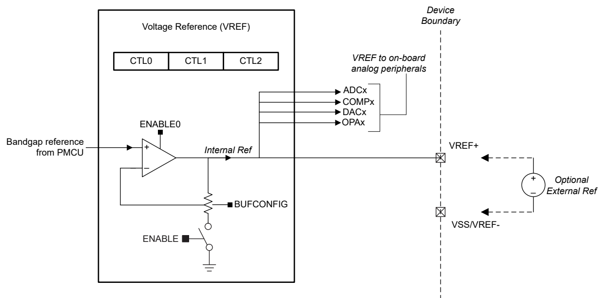
Figure 8-1. VREF Module
