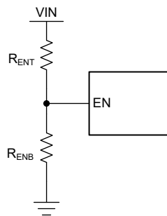
Figure 7-1. VIN UVLO Using the EN Pin
