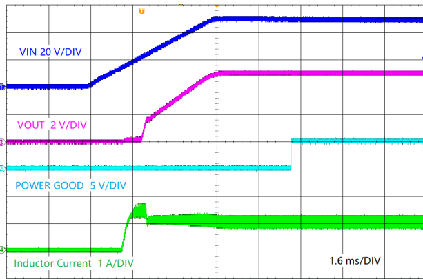
LMR38010-Q1 V_{OUT} = 5\text{ V} 400 kHz
