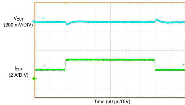
Figure 10-41. LMQ61460-Q1 Load Transient
