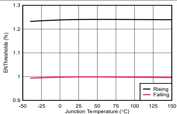
Figure 6-8. Enable UVLO
