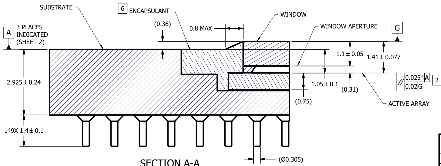
SECTION A-A SCALE 20 : 1
