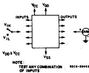
Fig. 14 - Input voltage.
