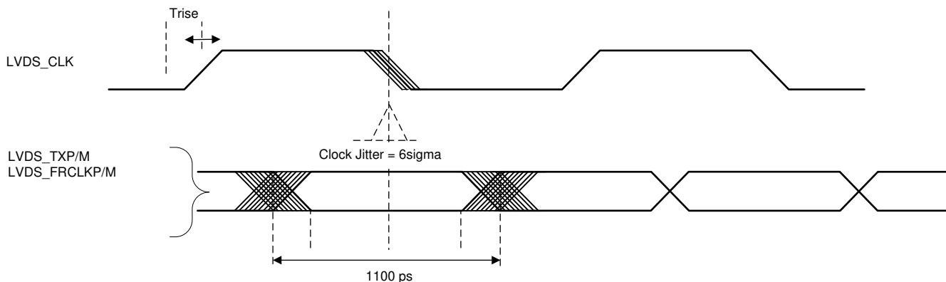
Figure 7-9. Timing Parameters
